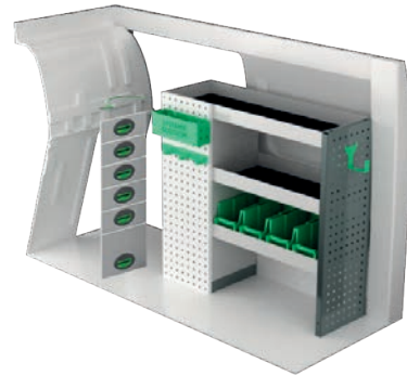
Tuotenro LxSxK Paino F43105 939x300x890 mm 41
