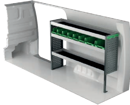
Tuotenro LxSxK Paino F42141 1453x300x1000 mm 28
