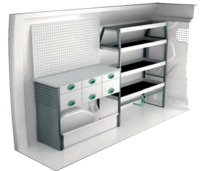
Tuotenro LxSxK Paino F41356 3053x300x1220 mm 115
