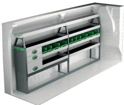
Tuotenro LxSxK Paino F49324 2446x300x1140 mm 67
