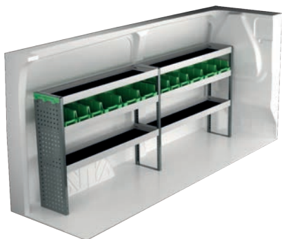
Tuotenro LxSxK Paino F49320 2446x300x1000 mm 44
